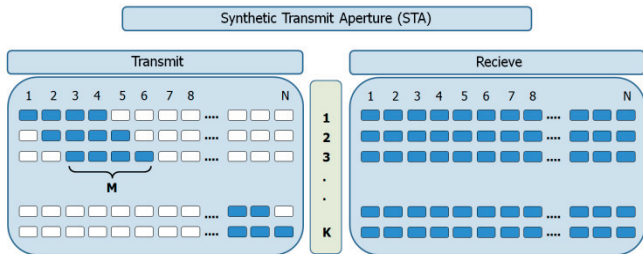
Fig.1. Scheme of STA mode
