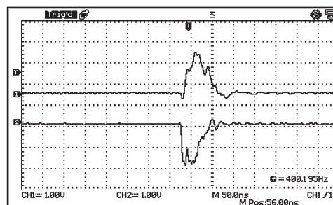
Rys. 3. Zobrazowanie przebiegów impulsu nadawczego (dolny) oraz impulsu odwróconego (górny) podawanego na wejście wyzwalające generatora sygnałowego Fig. 3. Display of the transmit pulse waveform (bottom) and the inverted pulse (top) of the signal generator triggering
