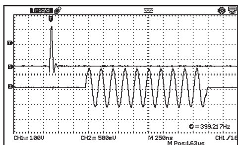
Rys. 4. Przebiegi typowych sygnałów z nadajnika defektoskopu (górnny) oraz sygnału testowego z generatora sygnałowego (dolny) Fig. 4. Waveforms of typical signals from the defectoscope transmitter (top) and test signal from the signal generator (bottom)
