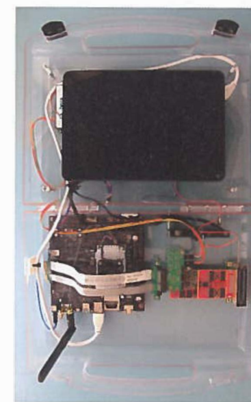
Rys. 1. Widok opracowanego demonstratora przenośnego systemu Phased-Array.
